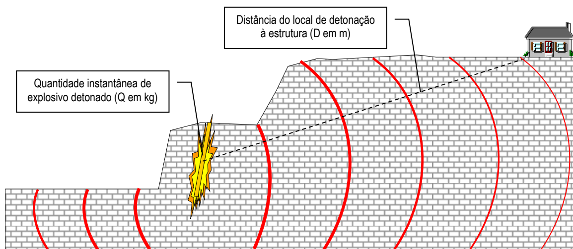
Figura III.36 – Perfil esquemático das principais variáveis que influenciam as vibrações.
