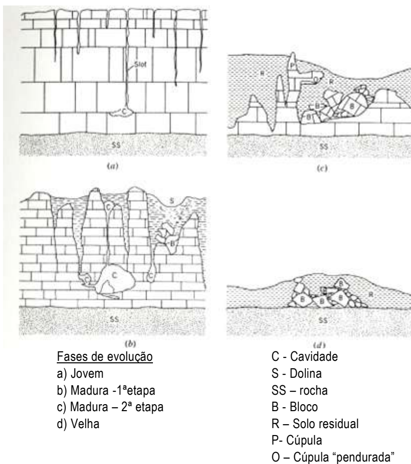
Figura III.7 - Fases de evolução da carsificação.
