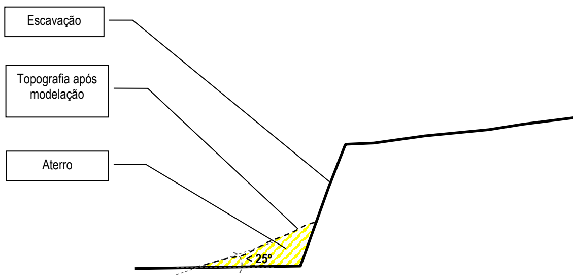
Figura II.10 – Perfil esquemático do aterro ao longo dos tardoze dos taludes de lavra.
