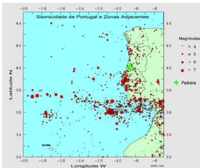
Figura III.13 – Sismicidade de Portugal e zonas adjacentes entre 33 a.C. e 1990 d.C.
