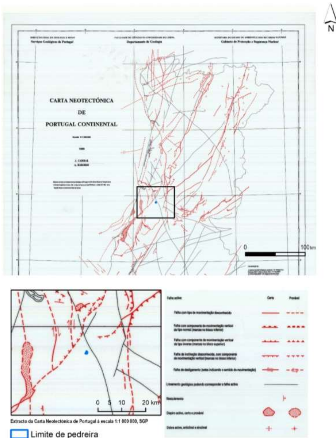
Figura III.12 – Carta Neotectónica de Portugal.
